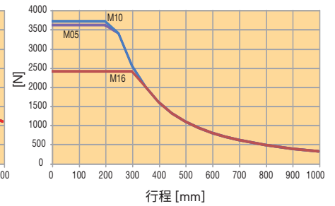
ETH032 - 安装方式 3
