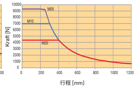
ETH050 - 安装方式 3
