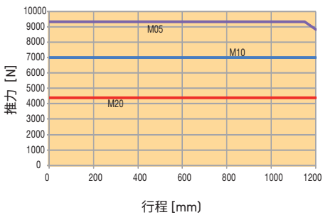
ETH050 - 安装方式 1
