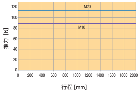
ETH125 - 安装方式 1
