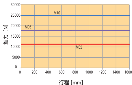
ETH080 - 安装方式 1
